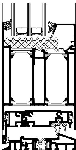
Profilsnitt sockelprofil
