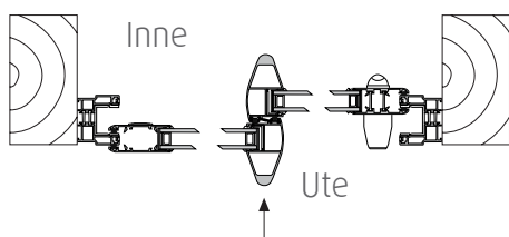
Thermo 2-delad skjutbar Spegelvänd utifrån sett
