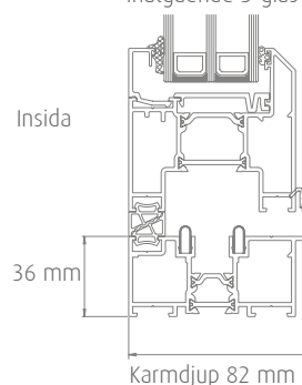
Inåtgående 3-glas
