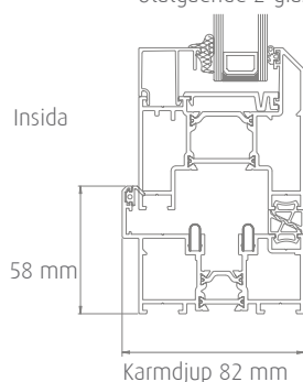
Utåtgående 2-glas
