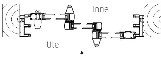
Thermo 3-delad skjutbar Spegelvänd utifrån sett
