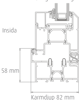
Utåtgående 2-glas
