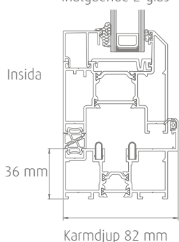
Inåtgående 2-glas
