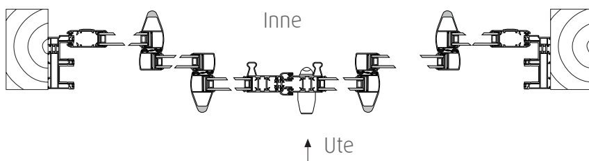
Thermo 6-delad skjutbar utifrån sett
