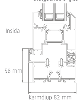
Utåtgående 3-glas
