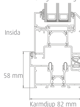
Utåtgående 3-glas
